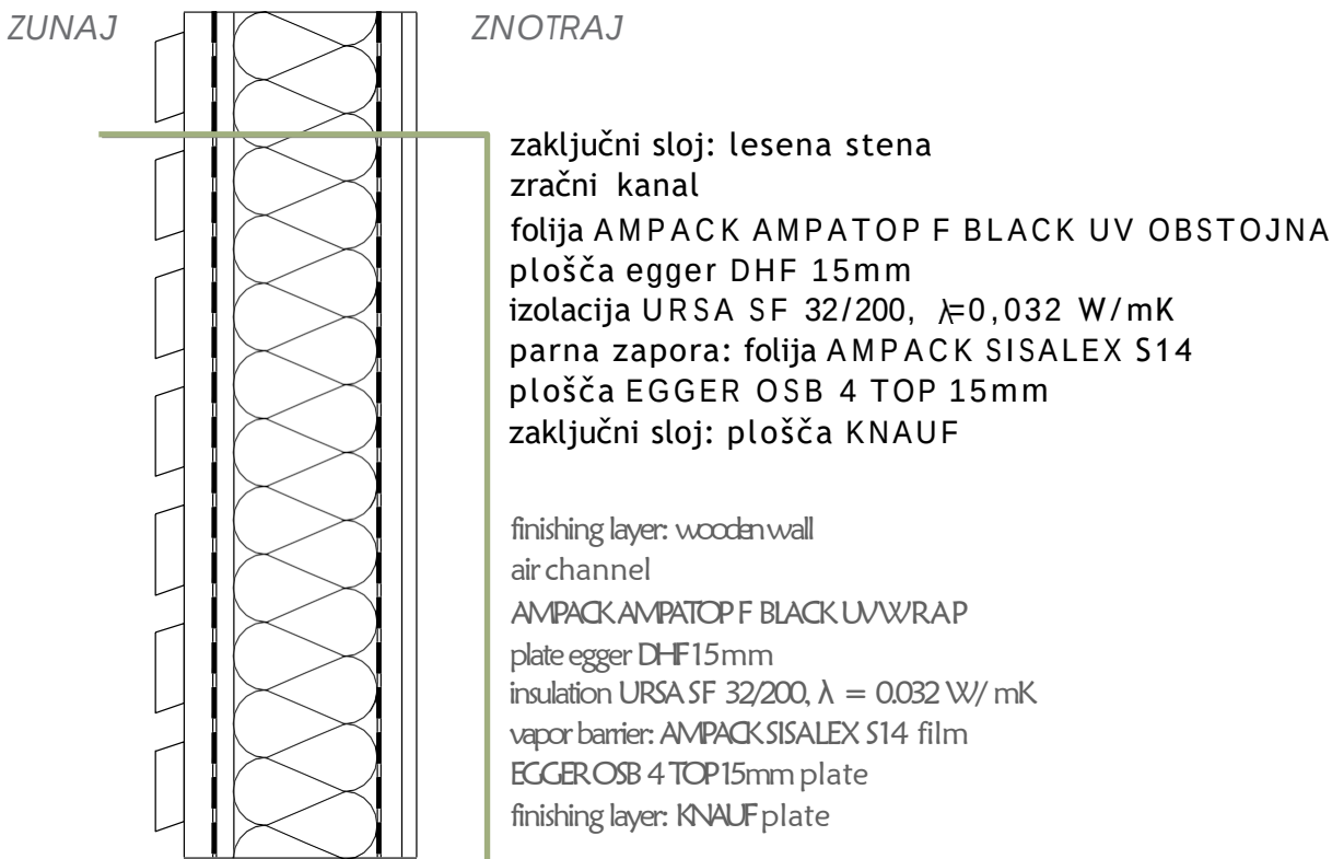
PREREZ STENE WALL SECTION
