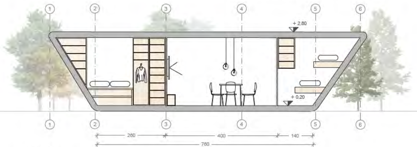
TLORIS M 1:75
